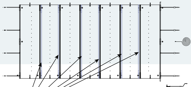
Platzieren Sie die Profile nebeneinander, um die Festigkeit der Abdeckung zu erhöhen und einen guten Abfluss des Regenwassers zu ermöglichen.
